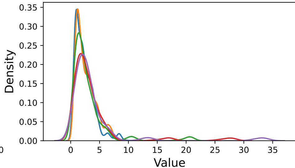
UOT
